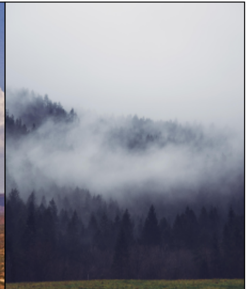
fog
